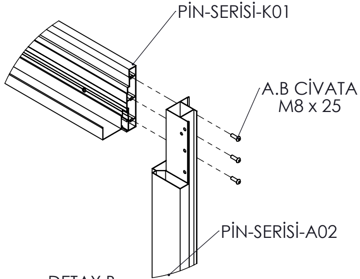
DETAY B ÖLÇEK 1 : 10
